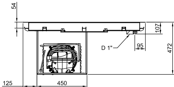
Lato posteriore
